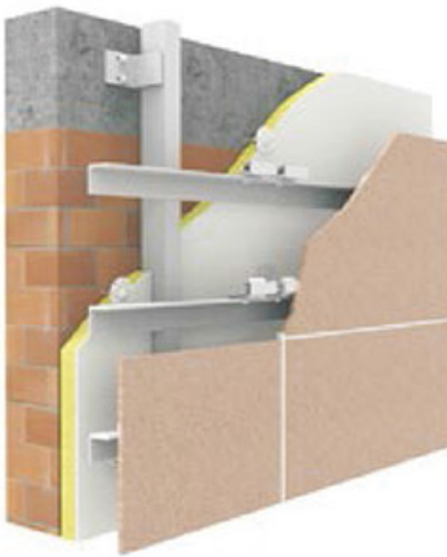
BACK SLOT TYPE L 背槽式L型 >>
